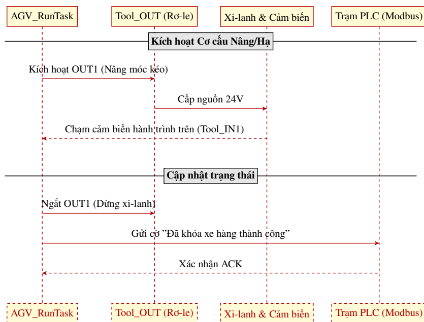
Hình 4.10 Sơ đồ tuần tự hoạt động của cơ cấu móc kéo xe hàng.
